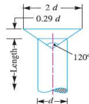
(d) Counter sunk head 120°.
